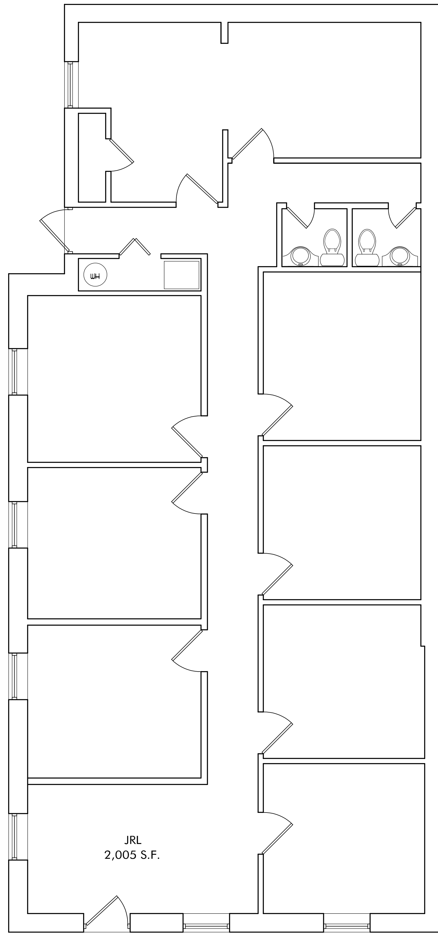
PLAN SCALE : 1/4"=1'-0"
