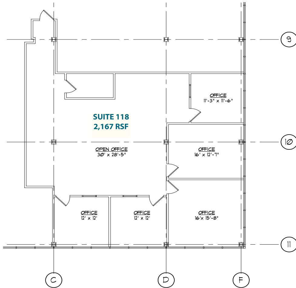
1 FIRST FLOOR PLAN L-1 | L-1 SCALE: 1/8"=1'-0"
