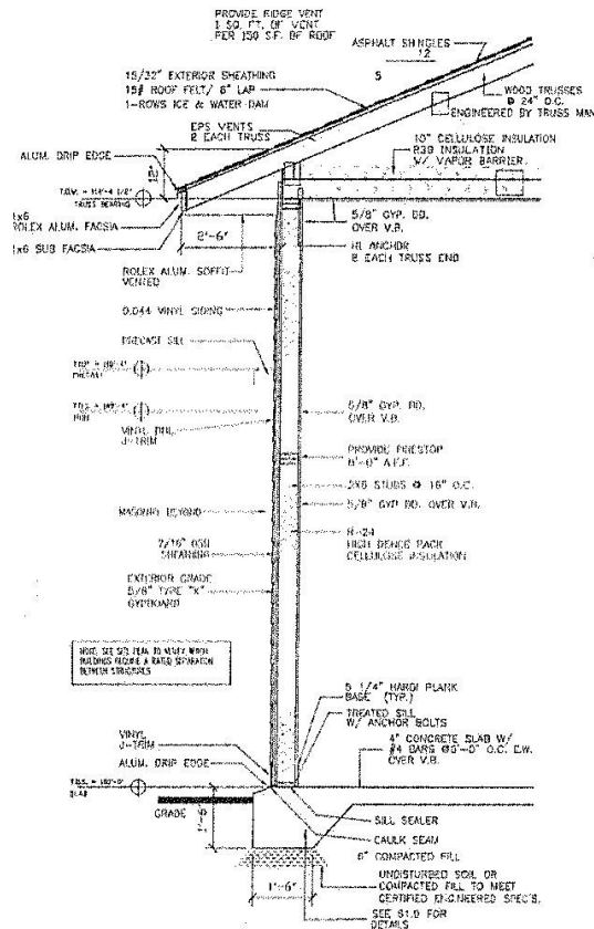
2 WALL SECTION SCALE: 1/2" = 1'-0"
