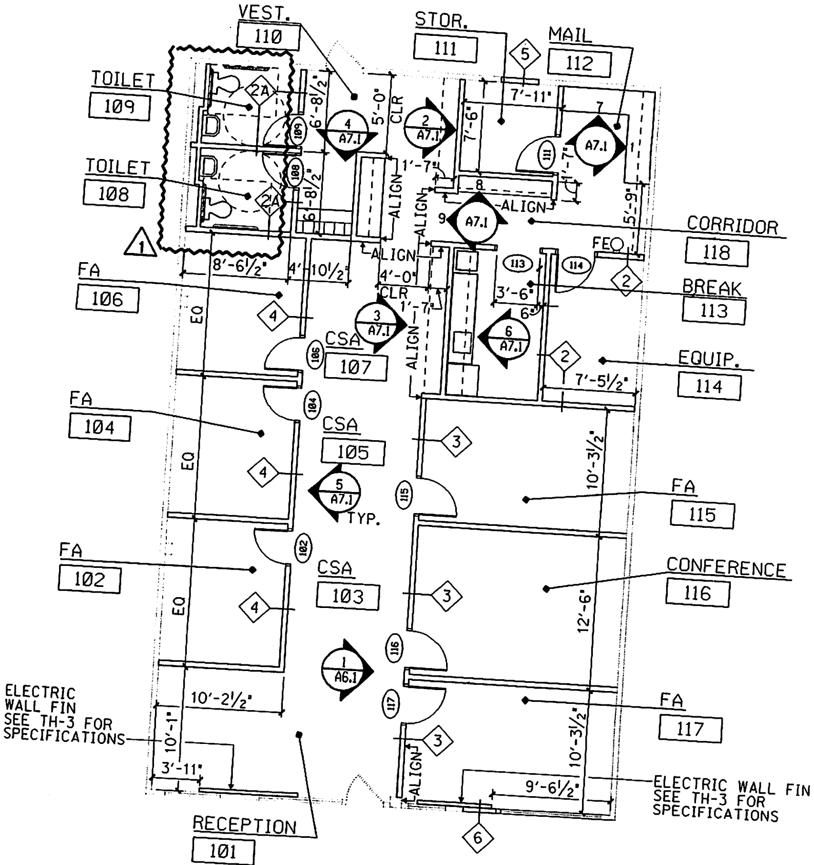
1 PARTITION PLAN A1.1 SCALE: 1/8" = 1'-0"
