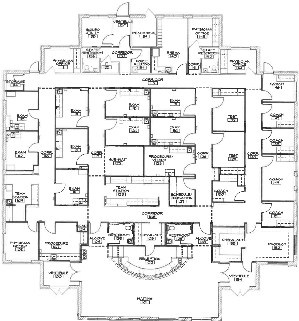
FLOOR PLAN 501 DUNLAP AVE. SAVOY, IL SCALE: N.T.S.
