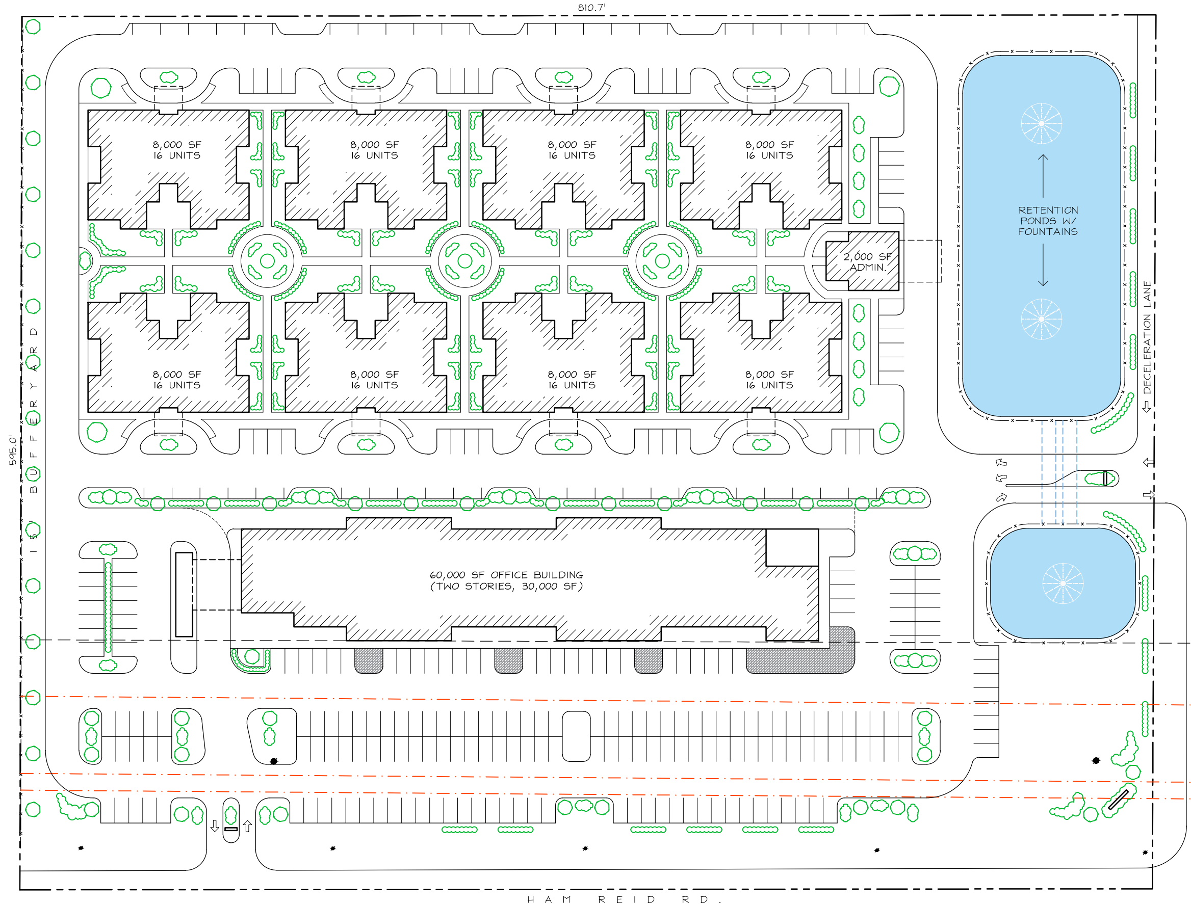
SITE PLAN SCALE: 1" = 70'
