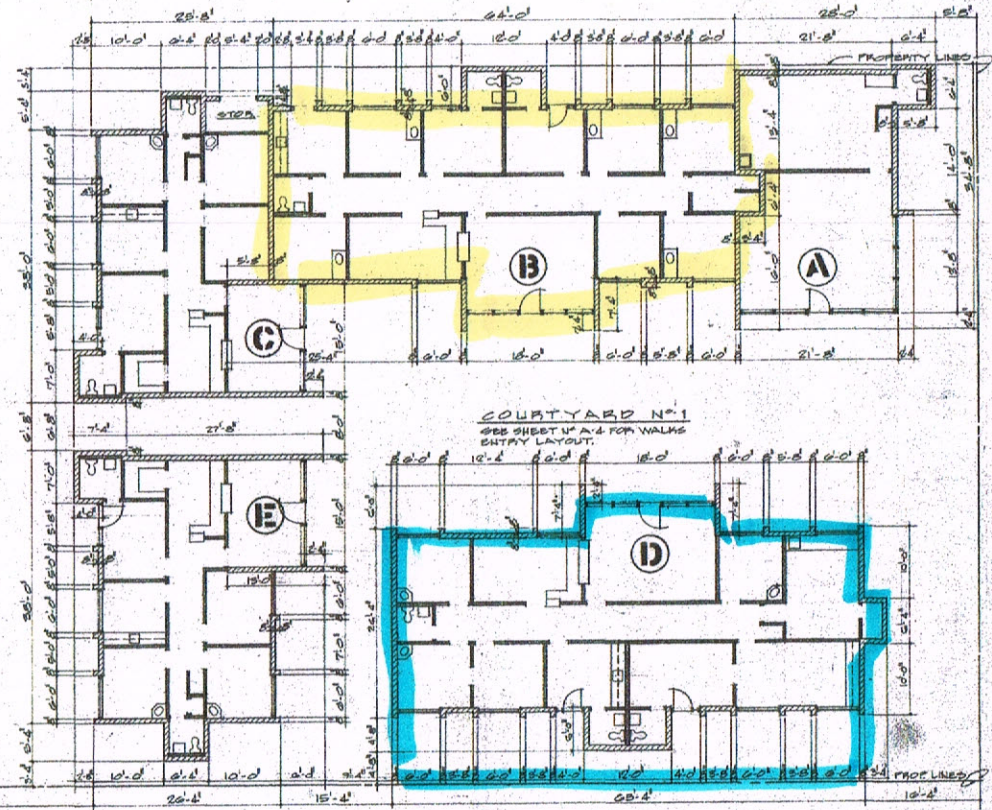
FLOOR PLAN N. 1/8" = 1'-0"
